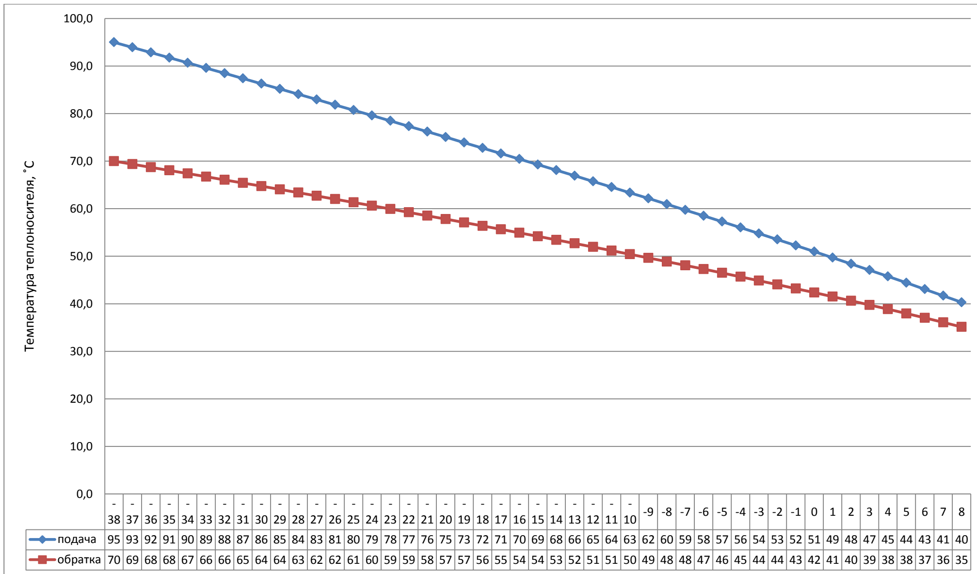
Рисунок 4.1 – Температурный график 95/70 °С
