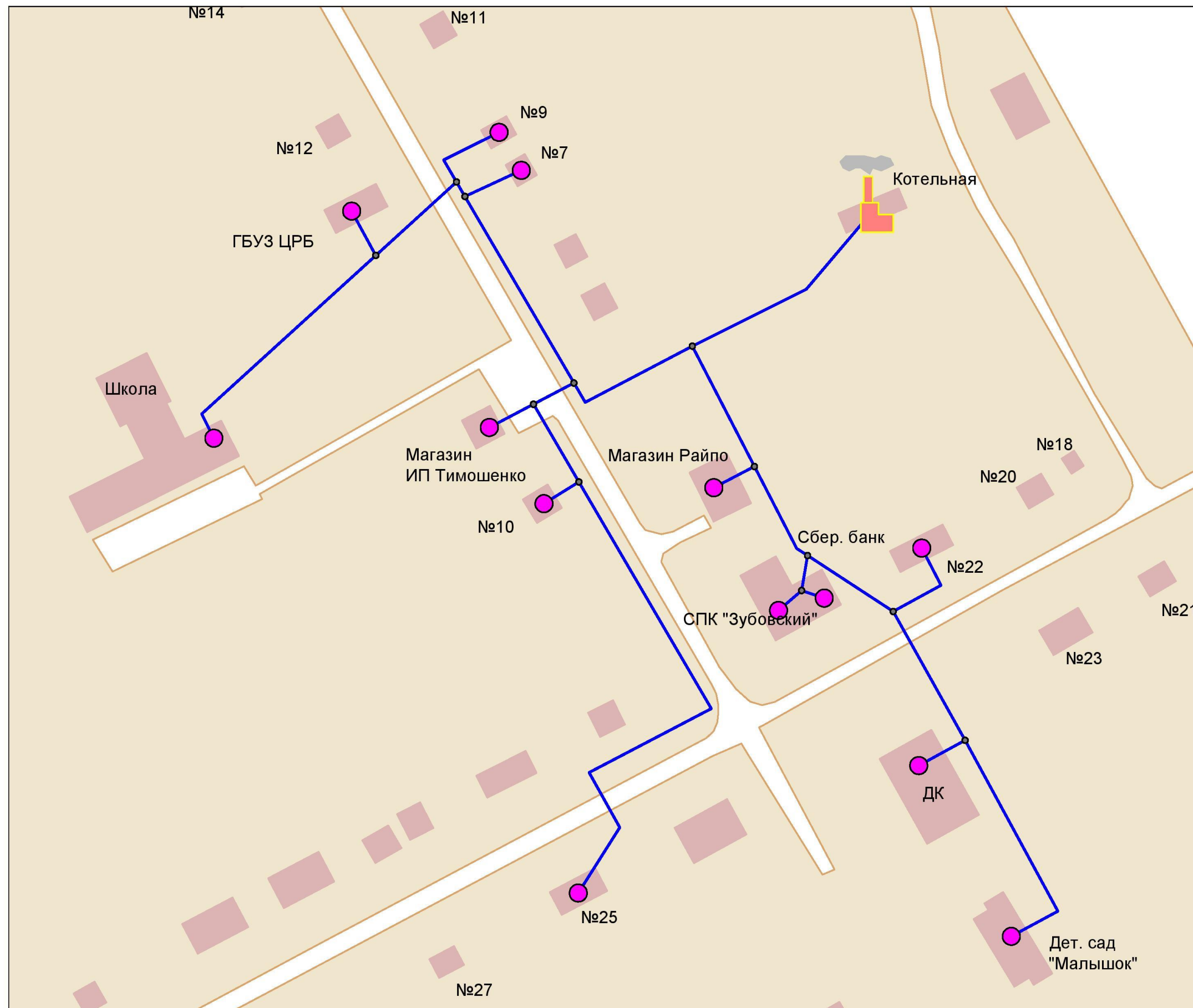
Рисунок 2.2 – Зона действия и схема тепловых сетей котельной с. Зубовка
