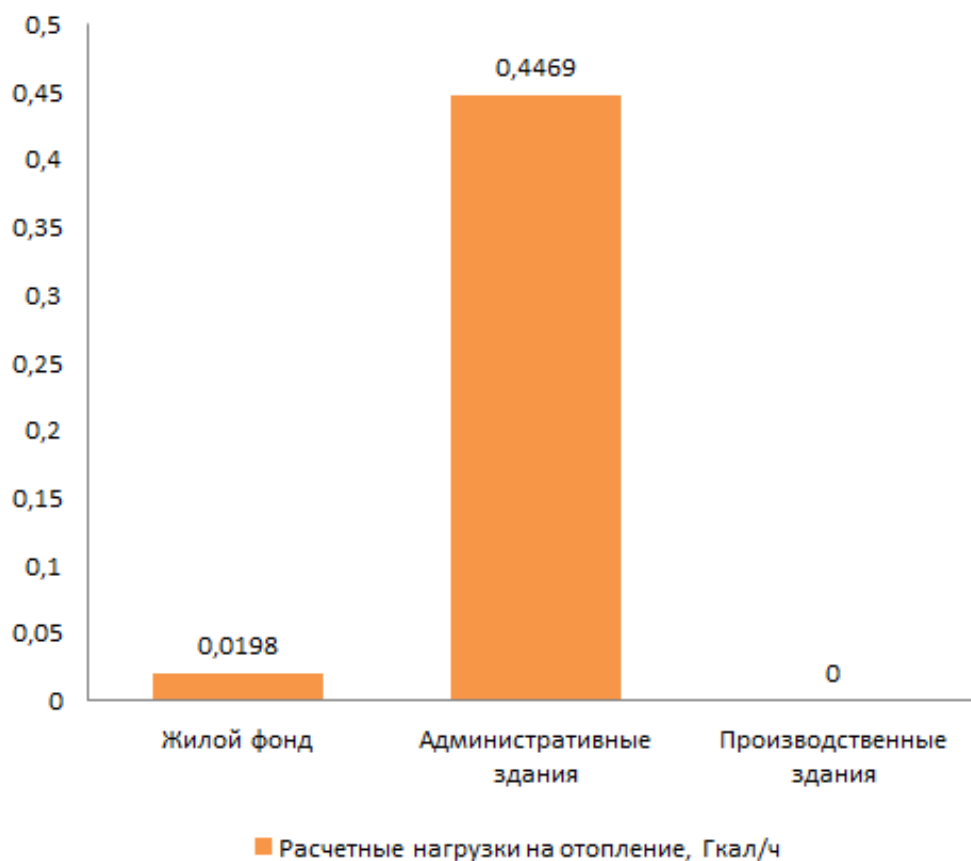
Рисунок 1.11 – Потребление тепловой энергии с. Zubovka с разбивкой по группам потребителей
