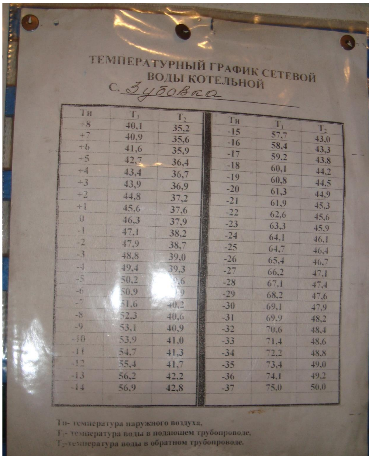
Рисунок 1.9 – Температурный график отпуска теплоносителя котельной с. Зубовка
