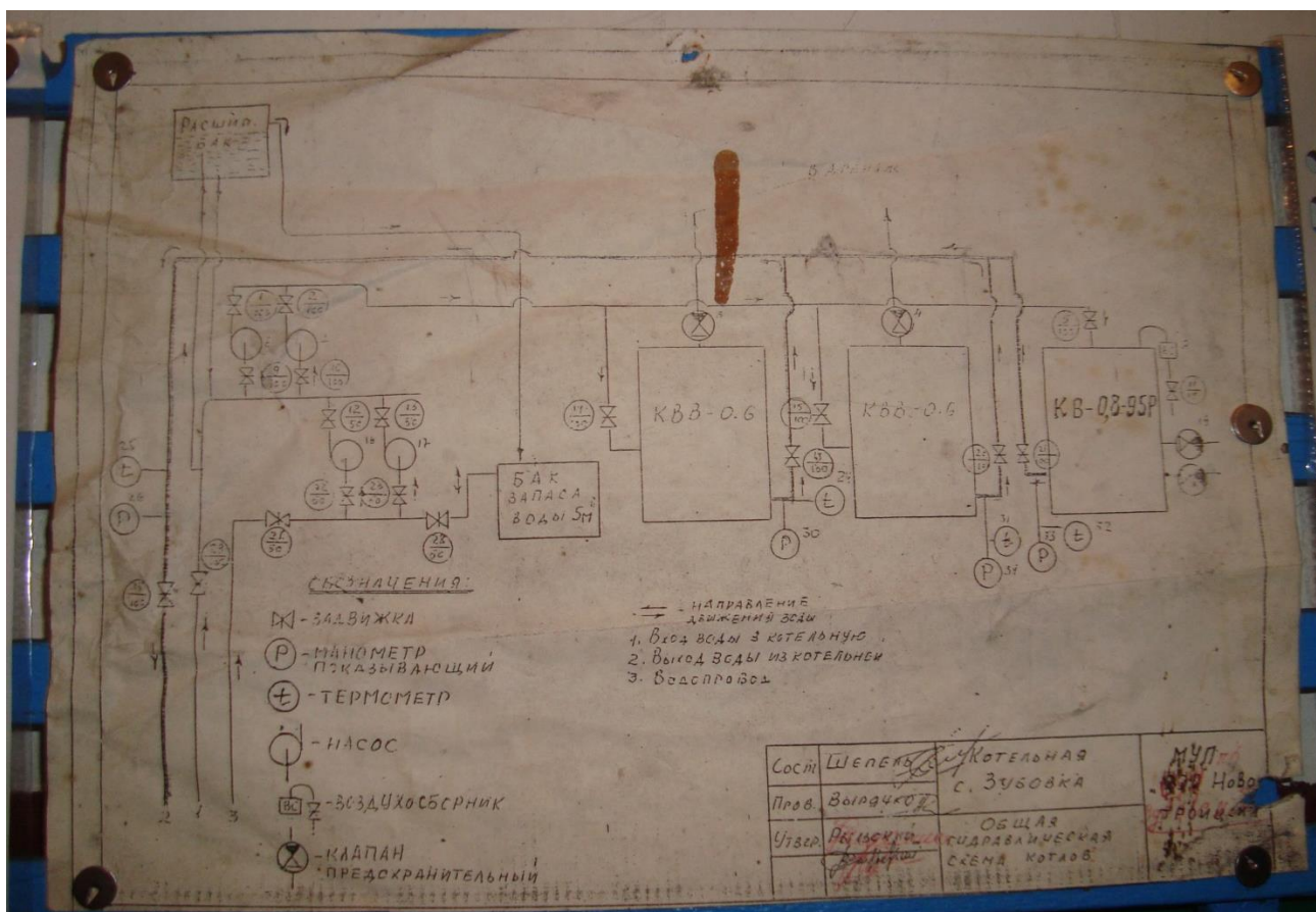
Рисунок 1.10 – Принципиальная схема котельной с. Zubovka
