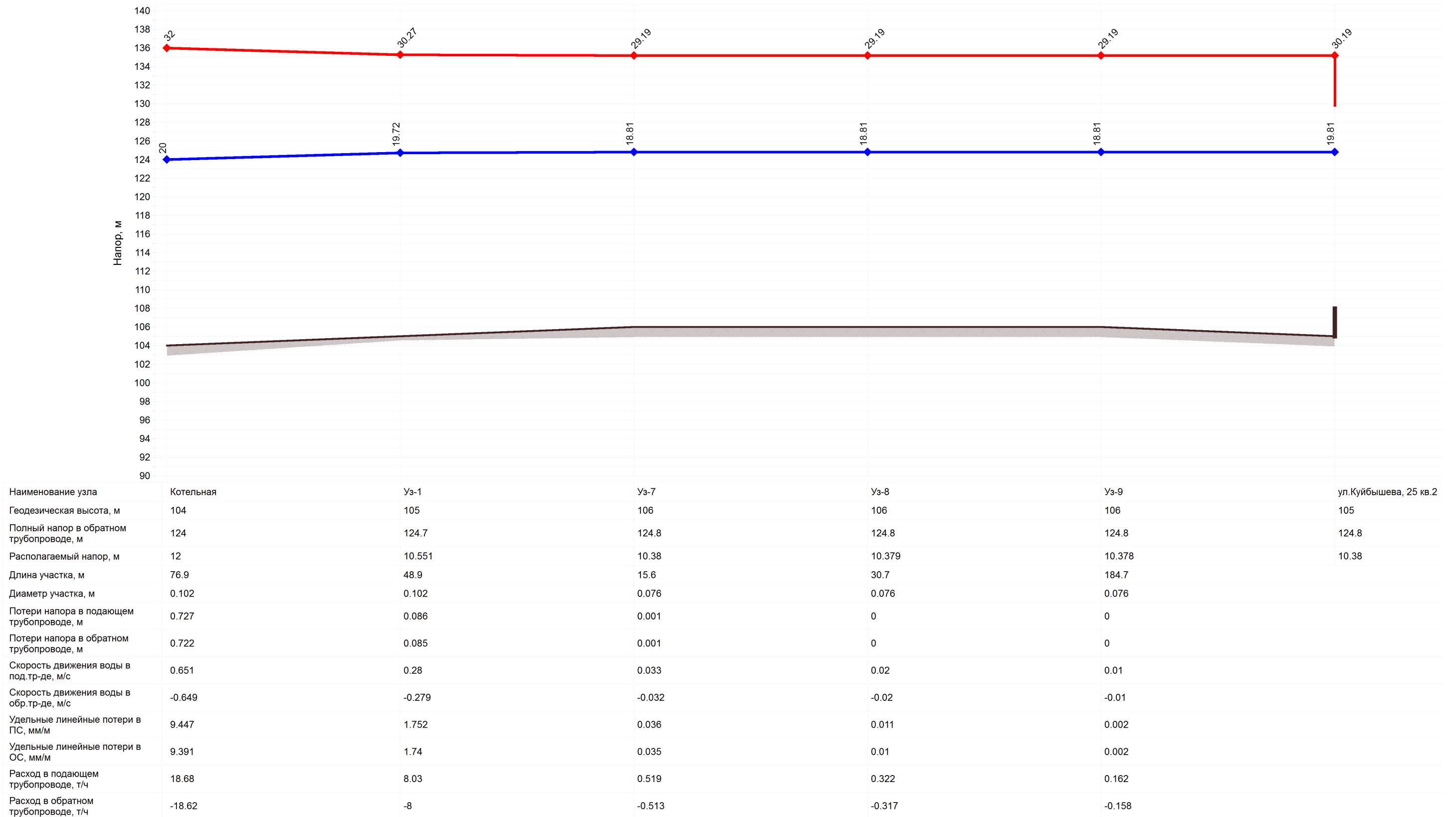
Рисунок 3.10 – Пьезометрический график участка сети от тепловой котельной до жилого здания №25 по ул. Куйбышева (существующий режим).
