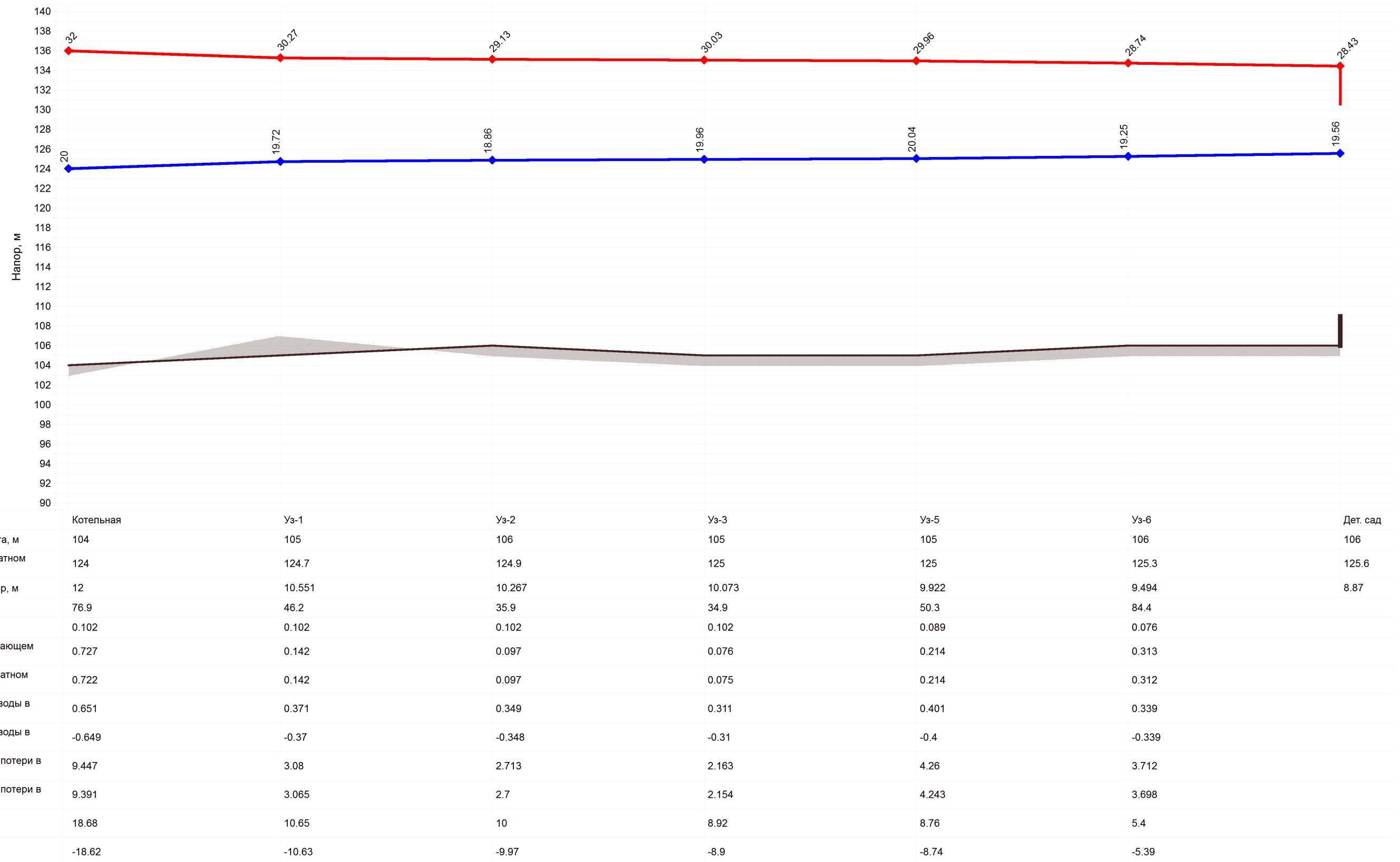
Рисунок 3.8 – Пьезометрический график участка тепловой сети от тепловой котельной до детского сада (существующий режим).
